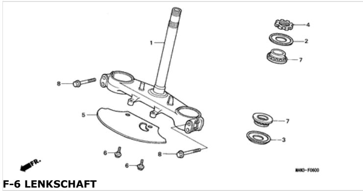
F-6 LENKSCHAFT
