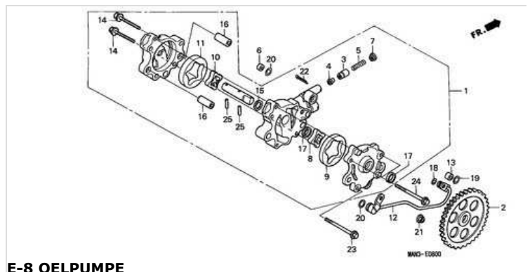
E-8 OELPUMPE
