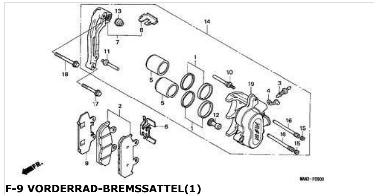
F-9 VORDERRAD-BREMSSATTEL(1)
