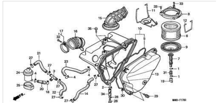
F-17 LUFTFILTER
