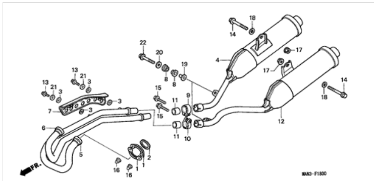
F-18 ABGAS-SCHALLDAEMPFER
