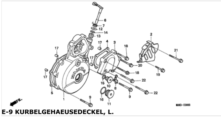
E-9 KURBELGEHAEUSEDECKEL, L.
