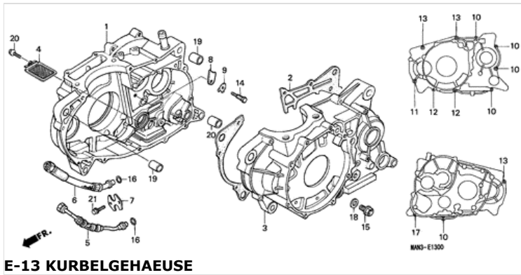
E-13 KURBELGEHAEUSE
