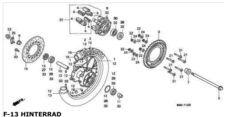
F-13 HINTERRAD
