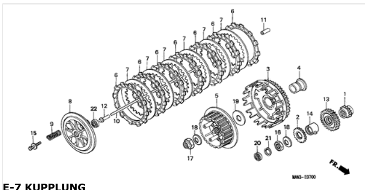
E-7 KUPPLUNG
