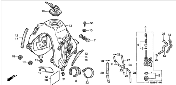
F-14 KRAFTSTOFFTANK
