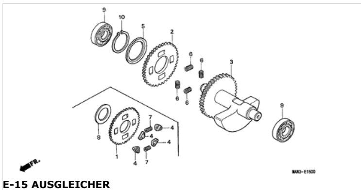
E-15 AUSGLEICHER
