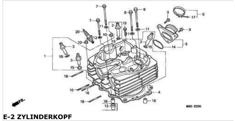
E-2 ZYLINDERKOPF
