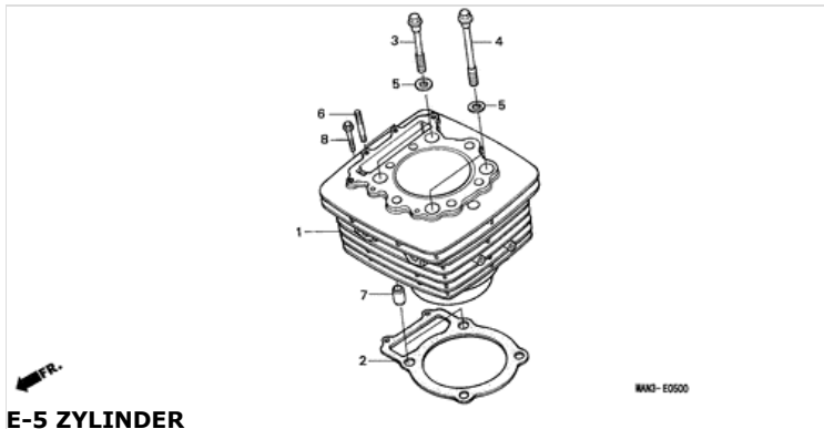
E-5 ZYLINDER
