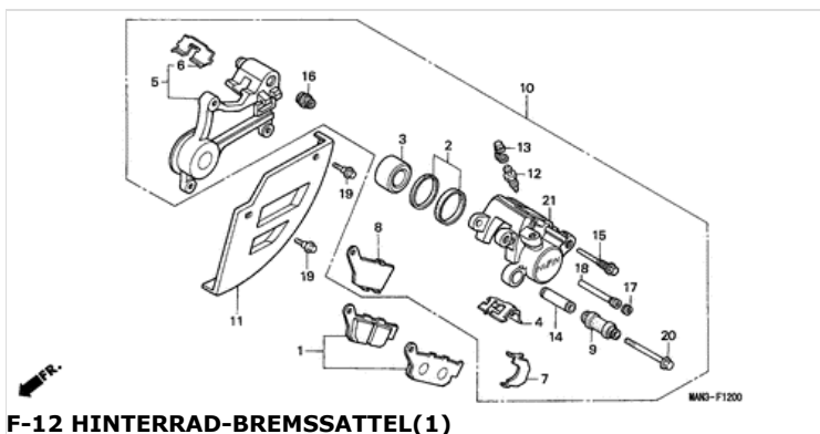
F-12 HINTERRAD-BREMSSATTEL(1)
