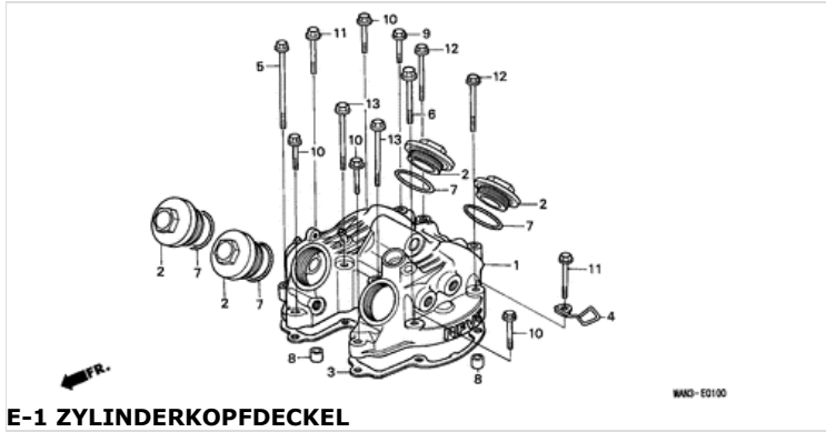
E-1 ZYLINDERKOPFDECKEL
