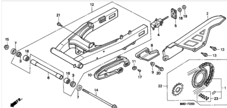
F-22 SCHWINGE
