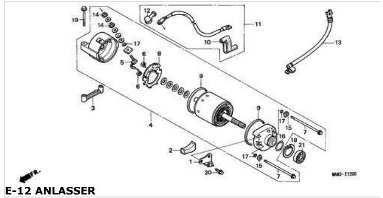
E-12 ANLASSER
