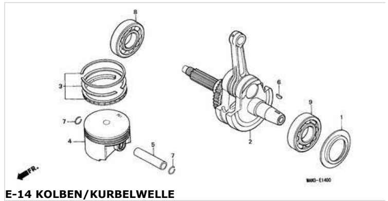
E-14 KOLBEN/KURBELWELLE
