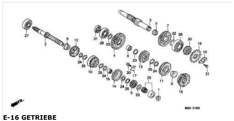
E-16 GETRIEBE
