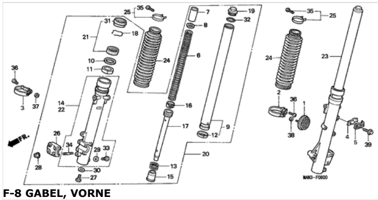
F-8 GABEL, VORNE
