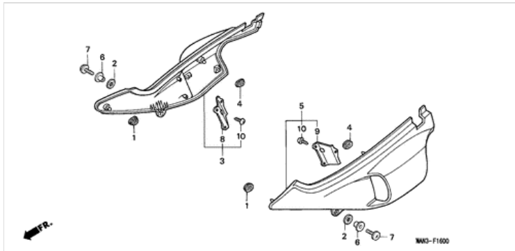
F-16 SEITENABDECKUNG(1)
