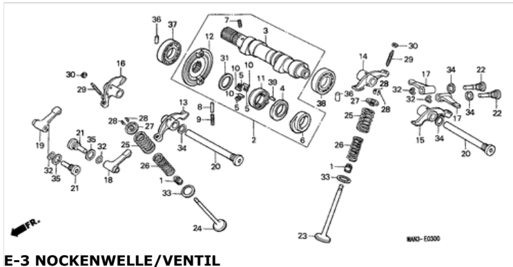
E-3 NOCKENWELLE/VENTIL
