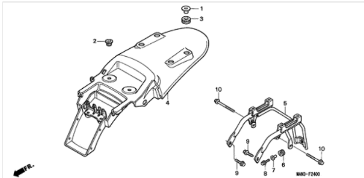
F-24 KOTFLUEGEL, HINTEN(1)
