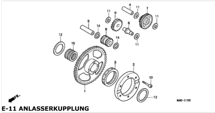
E-11 ANLASSERKUPPLUNG
