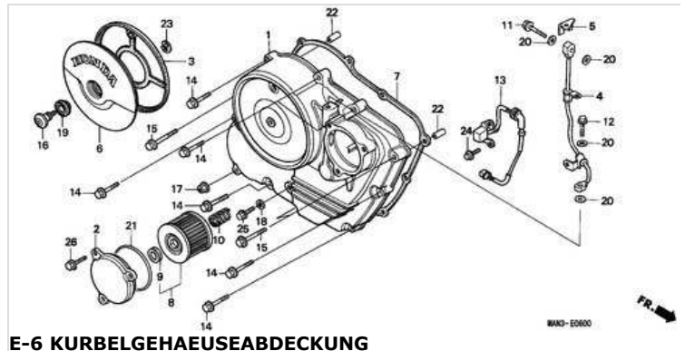
E-6 KURBELGEHAEUSEABDECKUNG
