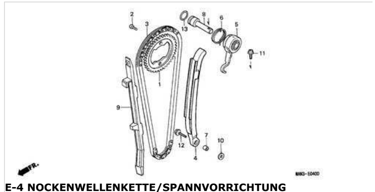
E-4 NOCKENWELLENKETTE/SPANNVORRICHTUNG
