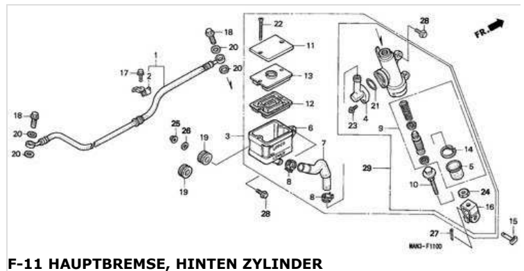
F-11 HAUPTBREMSE, HINTEN ZYLINDER
