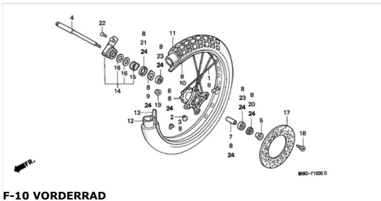
F-10 VORDERRAD
